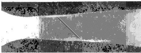
Рис. 225. Течение через сопло Лавая со скачком уплотнения ( p_2 < p_b ).
