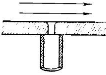
Рис. 48. Отверстие в стенке для измерения статического давления
