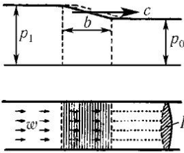
Рис. 209. Волна давления в трубе
