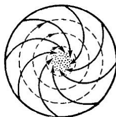
Рис. 114. Вторичный поток на дне круглого цилиндра
