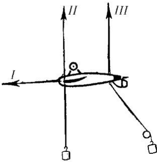
Рис. 207. Подвеска модели на трех проволоках
