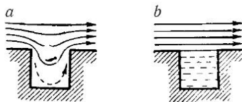
Рис. 47. Обтекание углубления в стенке
