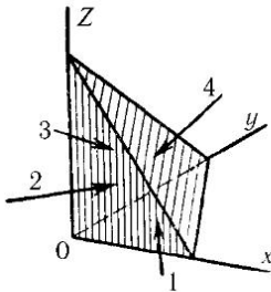
Рис. 3. Равновесие тетраэдра
