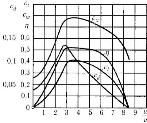
Рис. 181. Характеристики ветряка
