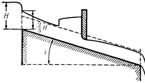
Рис. 139. Кривая подпора для i > i'
