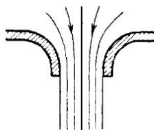
Рис. 32. Истечение из круглого отверстия с закругленными стенками
