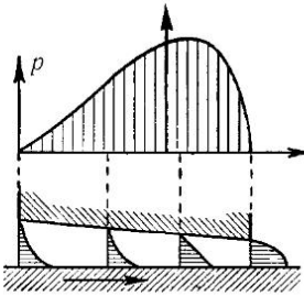
Рис. 123. Распределение давления под башмаком
