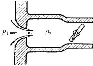
Рис. 219. Истечение сжатого воздуха из отверстия через дополнительную камеру с вентиляем
