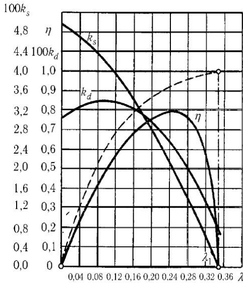
Рис. 180. Характеристики воздушного гребного винта
