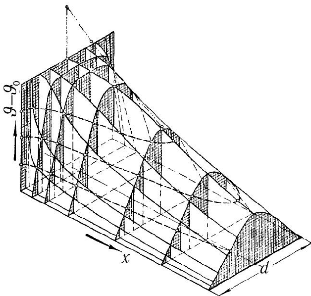
Рис. 307. Распределение температуры в трубе. Профили температур, вычерченные сплошными линиями, соответствуют значениям \frac{ax}{ud^2} = 0,005; 0,01; 0,02; 0,04; 0,06; 0,08 . Линия, вычерченная штрих-пунктиром, является графиком уравнения (99)
