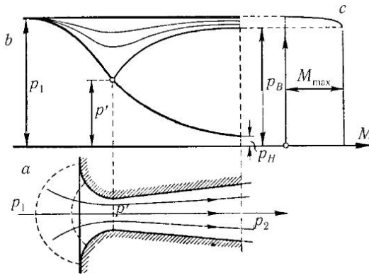
Рис. 220. Течение через сопло Лавали
