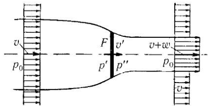
Рис. 176. Поле скоростей впереди и позади пропеллера
