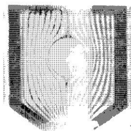
Рис. 120. Обтекание цилиндра в приборе Поля
