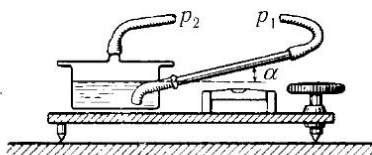
Рис. 14. Микроманометр Крелля
