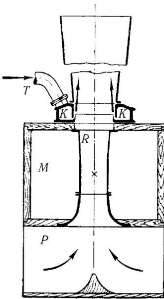
Рис. 257. Аэродинамическая труба высоких скоростей. Крестиком (x) отмечено место, где устанавливаются исследуемые модели. М — помещение для измерительных приборов
