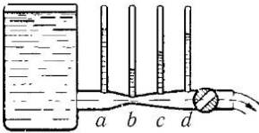
Рис. 52. Распределение давления в трубке с переменным сечением
