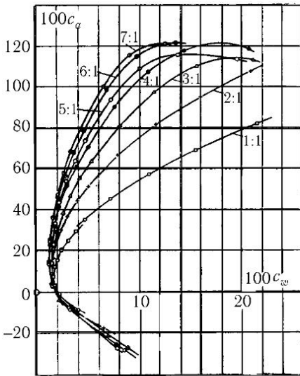
Рис. 170. Поляры для семи прямоугольных крыльев с различными относительными размахами. Числа для c_a и c_w увеличены в 100 раз
