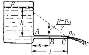
Рис. 37. Истечение из насадка
