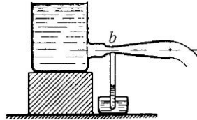
Рис. 53. Понижение давления в самом узком сечении трубы
