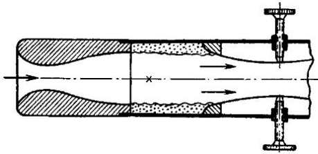
Рис. 259. Аэродинамическая труба сверхзвуковых скоростей
