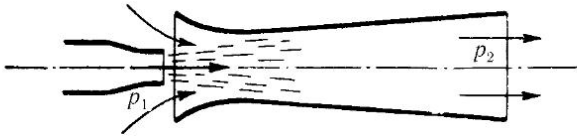
Рис. 134. Струйный насос
