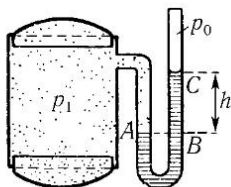
Рис. 11. Гидростатическое измерение давления (U-образная трубка)
