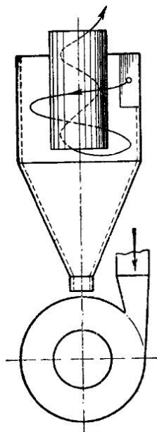
Рис. 282. Циклон
