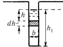
Рис. 136. Истечение через узкую щель
