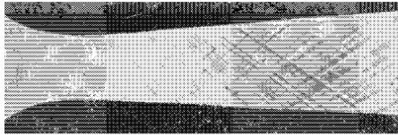
Рис. 223. Течение через сопло Лавая сжатого воздуха при начальном давлении в 7 ата и противодавлении в 1 ата . Скорость истечения — сверхзвуковая
