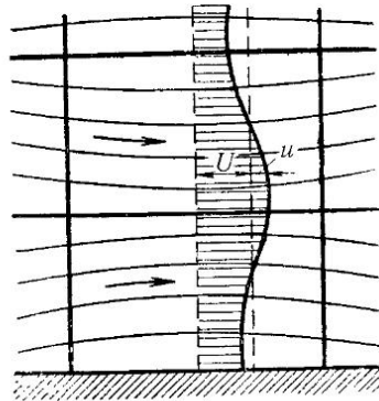
Рис. 299. Установившиеся волны
