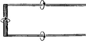
Рис. 166. Упрощенная система вихрей, заменяющих крыло
