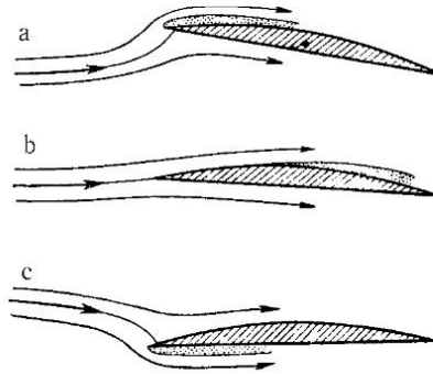
Рис. 266. Области возникновения кавитации на профиле
