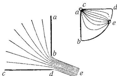
Рис. 60. Истечение через щель
