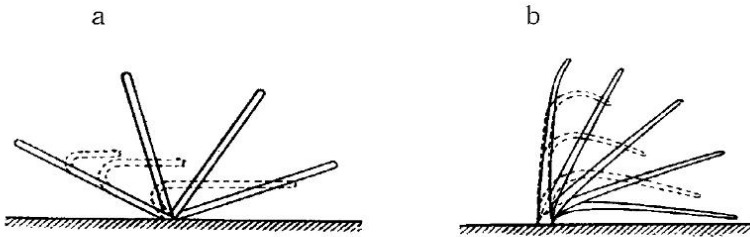
Рис. 185. Движение ресниц инфузорий
