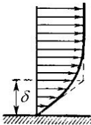
Рис. 92. Распределение скоростей вблизи стенки
