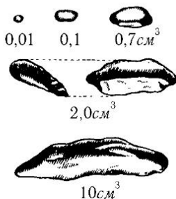
Рис. 280. Формы пузырьков воздуха, поднимающихся в воде (в 1/2 натуральной величины)
