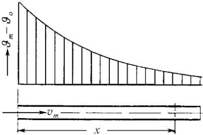
Рис. 306. Распределение разности температур \vartheta_m - \vartheta_0 вдоль трубы
