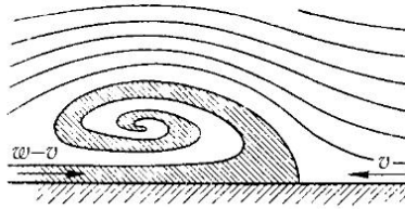
Рис. 295. Идеализированная картина продвижения фронта холодной массы воздуха (система отсчета движется вместе с фронтом)
