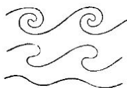
Рис. 41. Возникновение вихрей из волн на поверхности раздела
