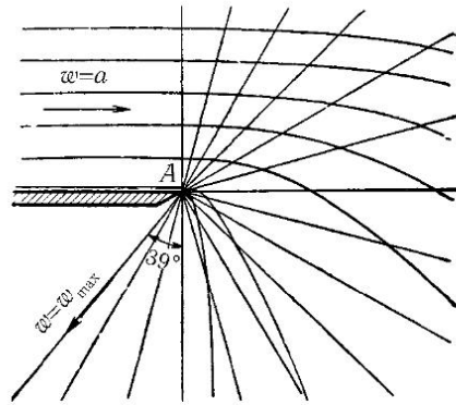
Рис. 230. Сверхзвуковой поток, движущийся в вакуум
