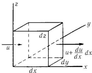
Рис. 27. К выводу уравнения неразрывности
