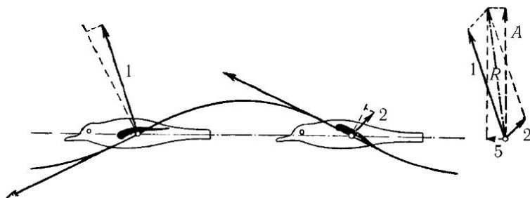
Рис. 183. Схема полета птиц, использующих свои крылья как весла
