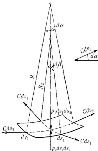
Рис. 20. Равновесие элементарной площадки на поверхности соприкосновения двух весомых жидкостей
