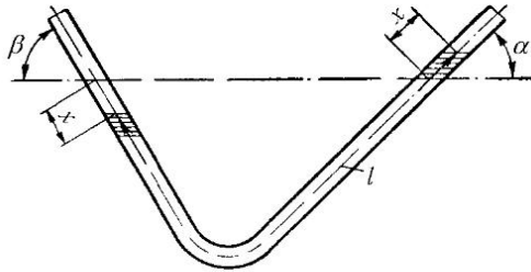
Рис. 38. Колебания столба жидкости
