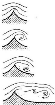
Рис. 44. Возникновение и распад поверхности раздела
