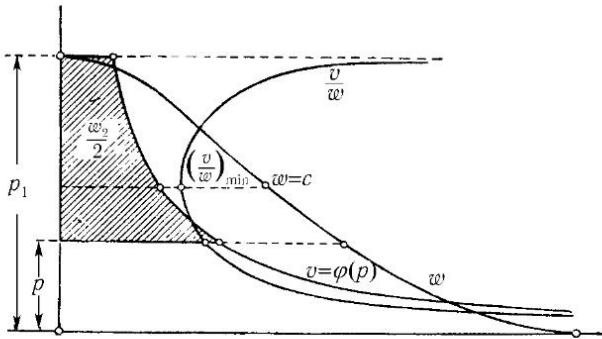
Рис. 215. Зависимость удельного объема v , скорости течения w и отношения \frac{v}{w} от давления p
