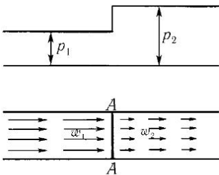
Рис. 221. Прямой скачок уплотнения
