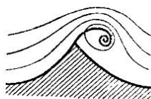
Рис. 43. Возникновение вихря при обтекании острого ребра
