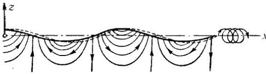
Рис. 81. Линии тока волнового движения
