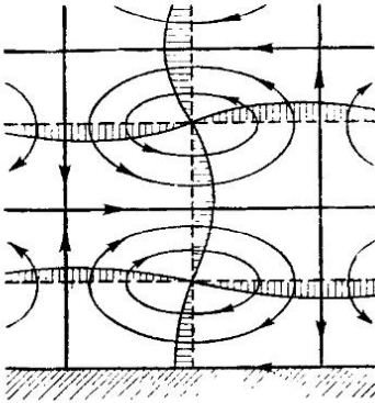
Рис. 298. Стоячие ячейковые волны гравитационного типа
