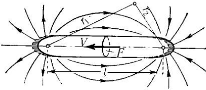
Рис. 56. Потенциальный поток около движущегося тела
