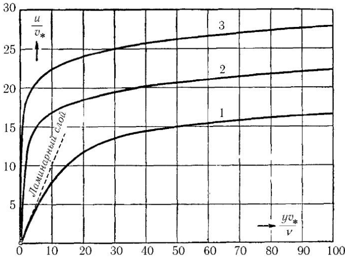
Рис. 100. Универсальный закон распределения скоростей
