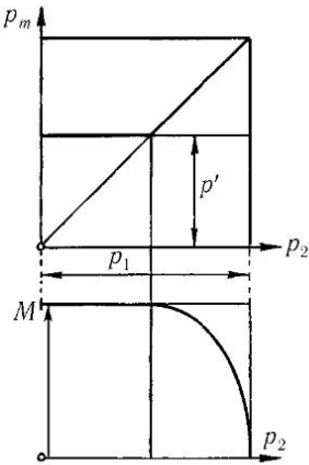
Рис. 218. Зависимость давления p_m и расхода M от противодействия p_2
