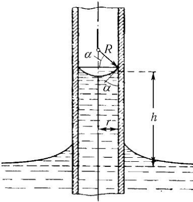
Рис. 24. Подъем жидкости в капиллярной трубке
