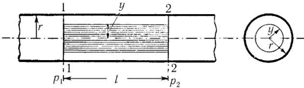
Рис. 91. Движение вязкой жидкости в трубе
