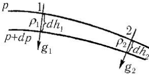
Рис. 18. Неоднородное силовое поле
