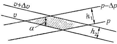
Рис. 297. Трубка, образованная пересечением поверхностей p = \text{const} и v = \text{const}
