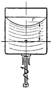
Рис. 19. Жидкость во вращающемся сосуде
