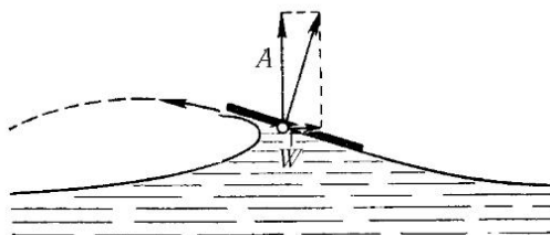
Рис. 273. Глссирование плоской пластинки с образованием струи
