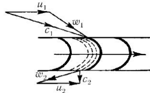
Рис. 186. План скоростей турбины равного давления
