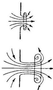
Рис. 45. Возникновение струи
