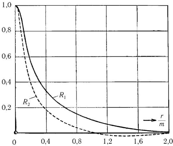
Рис. 103. Зависимость коэффициентов корреляции R_1 и R_2 от \frac{r}{m}
