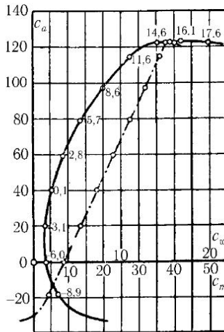
Рис. 161. Поляра (изображена сплошной линией) и моментная кривая (изображена штрихпунктиром). Для облегчения отсчета на осях абсцисс и ординат поставлены числа, в сто раз большие действительные значения C_a , C_w , и C_m
