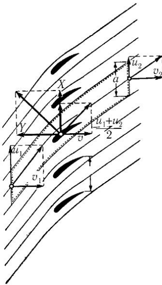
Рис. 78. Решетка из крыльев
