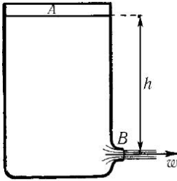
Рис. 30. Истечение из открытого сосуда
