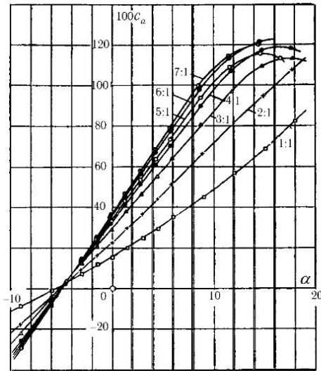
Рис. 173. Зависимость коэффициента подъемной силы прямоугольного крыла от угла атаки при различных относительных размахах. Числа для c_a на оси ординат увеличены в 100 раз
