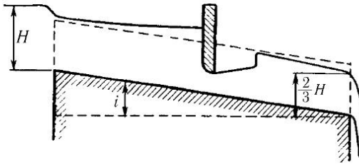
Рис. 138. Кривая подпора для i < i'
