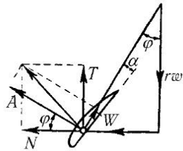
Рис. 177. Силы, действующие на элемент лопасти
