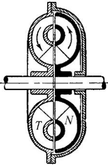
Рис. 197. Гидравлический привод: N — насос; T — турбина
