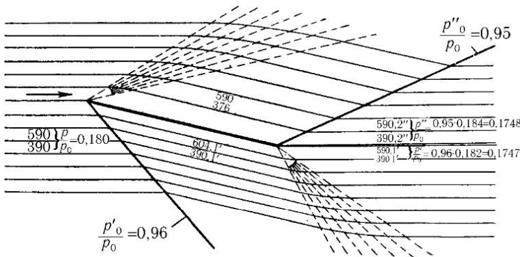
Рис. 254. Обтекание сверхзвуковым потоком наклоненной пластинки
