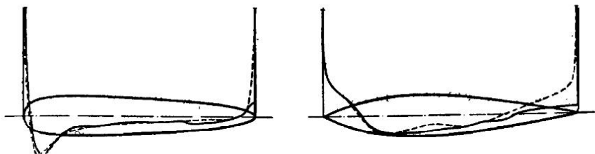
Рис. 151. Распределение давления на поверхности моделей дирижабля. Штрихами изображены вычисленные, а сплошными линиями — наблюдаемые распределения давления
