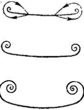
Рис. 46. Поверхность раздела позади наклоненной пластинки
