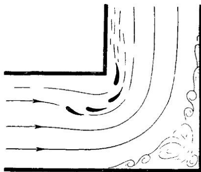
Рис. 112. Поворотные лопатки в канале.
