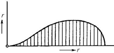
Рис. 179. Распределение циркуляции вдоль радиуса лопасти
