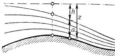
Рис. 85. Перетекание воды через плотину
