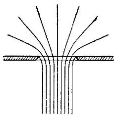
Рис. 31. Истечение из круглого отверстия в тонкой стенке
