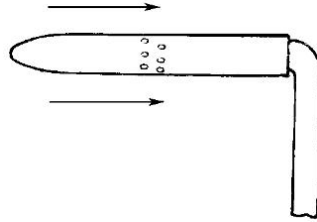
Рис. 50. Зонд для измерения статического давления (нифер)
