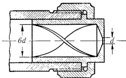
Рис. 279. Жиклер для распыления горючего
