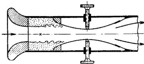
Рис. 258. Аэродинамическая труба дозвуковых скоростей
