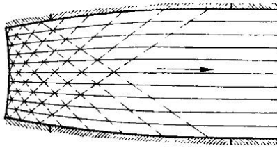
Рис. 241. Насадок для получения параллельной струи
