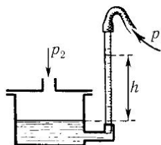
Рис. 12. Жидкостный манометр
