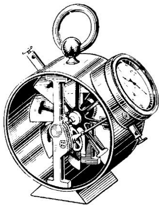
Рис. 202. Крыльчатый анемометр
