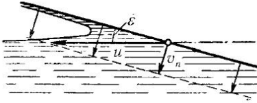
Рис. 270. Опускание на воду пластинки с нормальной скоростью v_n
