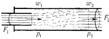
Рис. 77. Внезапное расширение трубы
