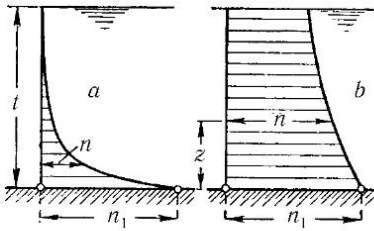
Рис. 284. Распределение взвешенных частиц в потоке
