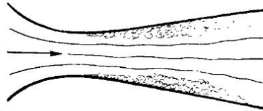
Рис. 262. Область, охватываемая кавитацией при малом противо-давлении
