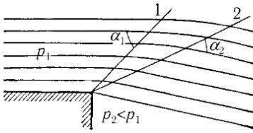
Рис. 231. Линии разрежения
