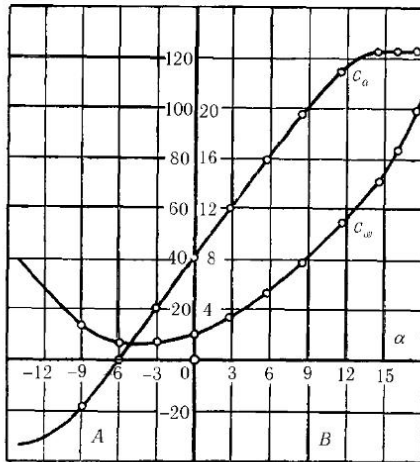
Рис. 158. Зависимость коэффициентов подъемной силы ( c_a ) и лобового сопротивления ( c_w ) от угла атаки \alpha . Для облегчения отсчета на оси ординат поставлены числа, в сто раз больше действительных значений c_a и c_w
