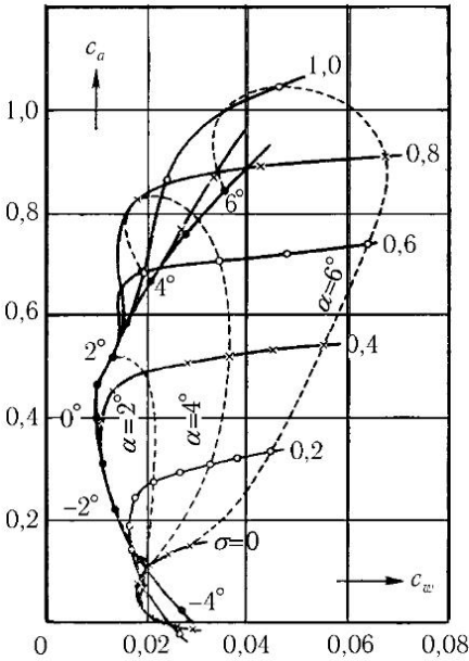
Рис. 264. Кавитационные поляры
