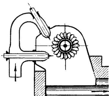
Рис. 190. Схема установки колеса Пельтона; слева — два сопла
