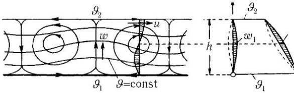
Рис. 315. Конвективный поток
