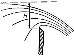
Рис. 135. Водослив через плотину с острой вершиной
