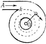
Рис. 36. Течение в спиральной камере
