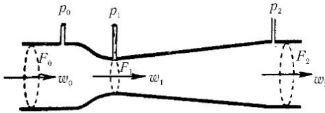
Рис. 133. Трубка Вентури
