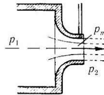
Рис. 217. Измерение давления в выходном сечении
