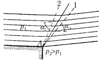
Рис. 233. Косой скачок уплотнения
