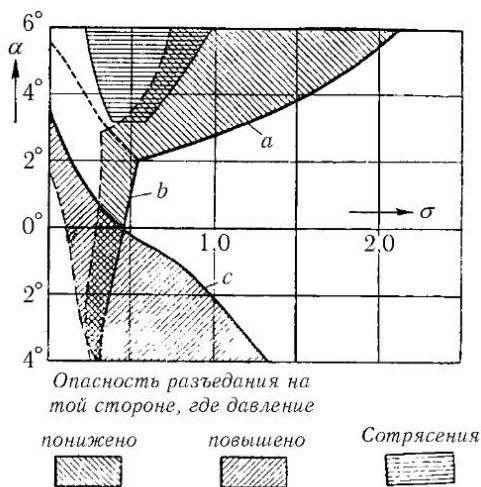
Рис. 265. Кавитационная диаграмма
