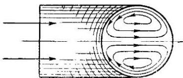
Рис. 113. Вторичные потоки в округлой изогнутой трубе
