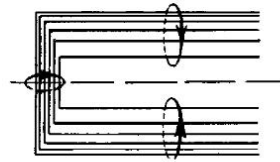
Рис. 167. Уточненная система вихрей, заменяющих крыло
