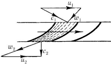
Рис. 187. План скоростей турбины избыточного давления
