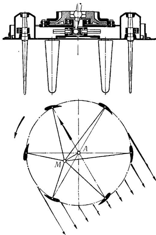
Рис. 182. Пропеллер Фохта – Шнейдера
