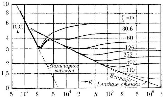
Рис. 128. Зависимость коэффициента сопротивления \lambda от числа Рейнольдса (сплошные кривые — по измерениям Никурадзе, штрихпунктирная кривая — по измерениям Бауэра и Галавича)
