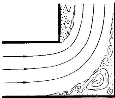
Рис. 105. Поток в прямоугольном колене
