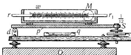
Рис. 15. Манометрический уровень Теплера
