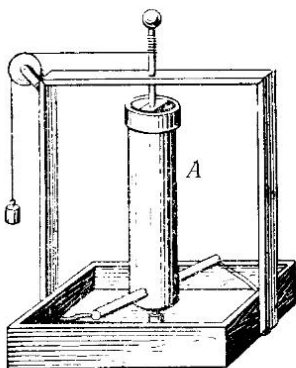
Рис. 75. Колесо Сегнера
