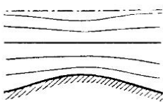
Рис. 87. Профиль свободной поверхности воды при перетекании через возвышение на дне русла. Скорость течения меньше критической скорости \sqrt{gh}
