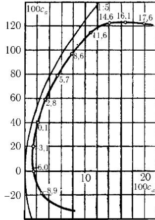
Рис. 172. Парабола индуктивного сопротивления
