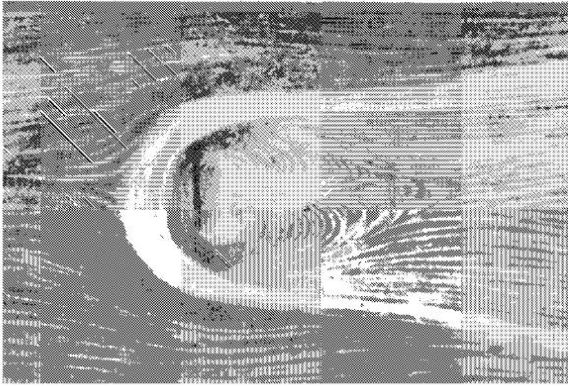
Рис. 115. Вторичный поток на дне круглого цилиндра
