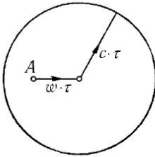
Рис. 210. Волна давления при скорости течения, меньшей скорости звука
