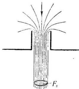
Рис. 76. Насадок Борда
