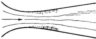
Рис. 261. Область, охватываемая кавитацией при большом противо-давлении
