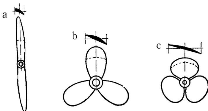
Рис. 178. а) воздушный винт; б) тихоходный водяной винт; в) быстроходный водяной винт
