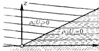
Рис. 302. Поверхность раздела между теплым и холодным потоками
