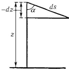
Рис. 29. К выводу уравнения Бернулли
