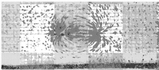
Рис. 121. Движение жидкости около источника и стока
