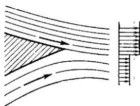
Рис. 39. Слияние двух потоков
