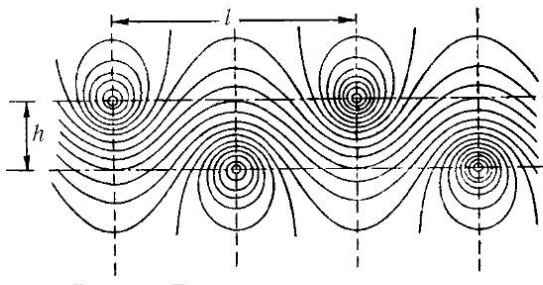
Рис. 144. Линии тока в вихревой дорожке
