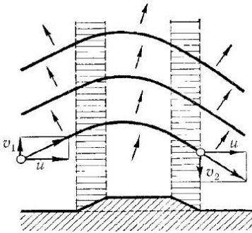
Рис. 288. Обтекание гребня горы
