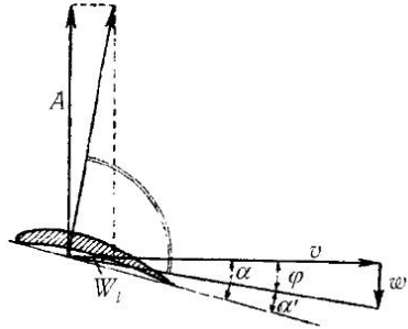
Рис. 165. Возникновение индуктивного сопротивления
