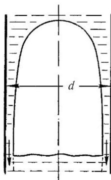
Рис. 281. Пузырь воздуха в вертикальной трубе
