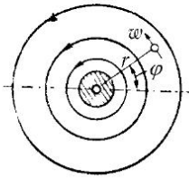
Рис. 61. Потенциальный поток с циркуляцией
