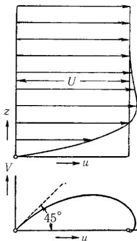
Рис. 289. Ламинарное приземное течение
