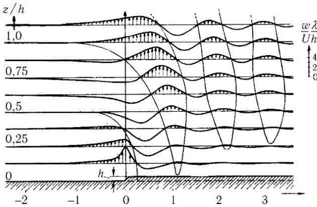
Рис. 301. Волны над краем плоскогорья
