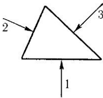
Рис. 4. Силы, действующие на боковые грани призмы
