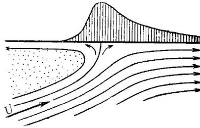
Рис. 271. Линии тока течения около пластинки, опускающейся на воду с нормальной скоростью v_n , в системе отсчета, движущейся вправо со скоростью U = \frac{v_n}{\sin \alpha}
