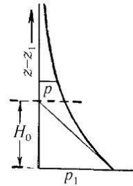
Рис. 10. Распределение давления в атмосфере с постоянной по высоте температурой
