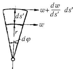
Рис. 54. Четырехугольник, вдоль которого вычисляется циркуляция
