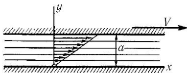
Рис. 90. Движение вязкой жидкости между двумя пластинками
