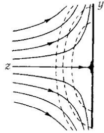
Рис. 55. Трехмерный симметричный относительно оси поток перед пластинкой
