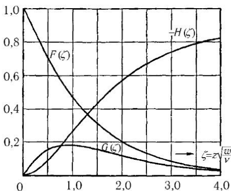
Рис. 292. Вращающийся диск в покоящейся жидкости
