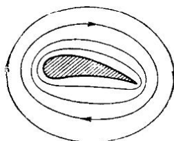
Рис. 65. Циркуляционный поток вокруг крыла
