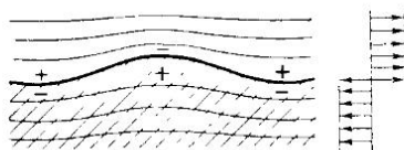
Рис. 40. Возникновение волн на поверхности раздела
