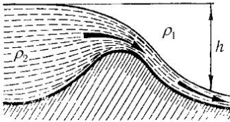
Рис. 294. Вторжение холодного воздуха в горах
