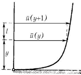
Рис. 95. К выводу формулы для дополнительного касательного напряжения
