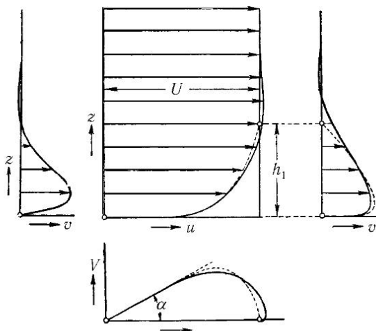
Рис. 290. Турбулентное приземное течение
