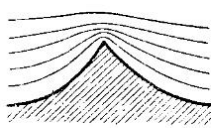
Рис. 42. Обтекание острого ребра
