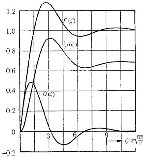
Рис. 293. Вращающаяся жидкость на покоящемся основании
