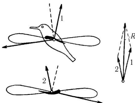
Рис. 184. Схема полета птиц, использующих свои крылья как геликоптер
