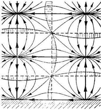
Рис. 300. Стоячие ячейковые волны звукового типа
