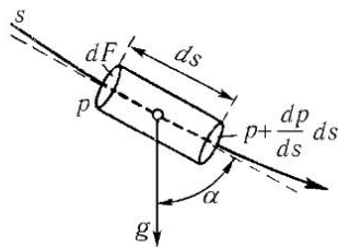
Рис. 28. К выводу уравнения Бернулли
