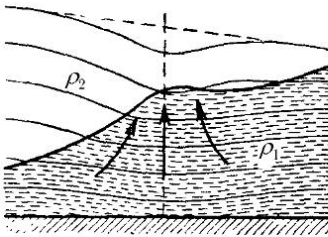
Рис. 303. Область низкого давления, вызванная вихрем в стратосфере
