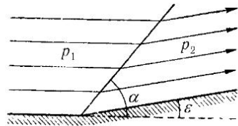
Рис. 255. К вычислению распределения давления в сверхзвуковом потоке
