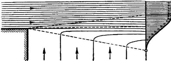
Рис. 97. Разрыв края струи
