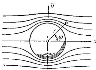
Рис. 58. Потенциальный поток около шара
