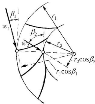
Рис. 79. К выводу теоремы Эйлера о турбине
