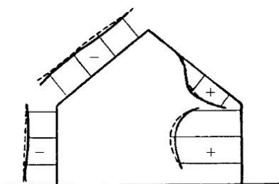
Рис. 147. Давление ветра на стены и крышу здания
