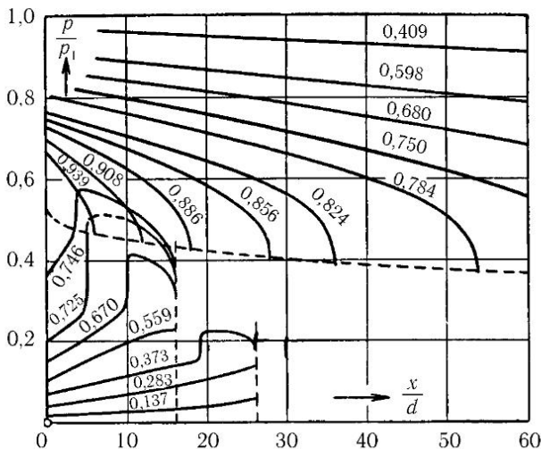
Рис. 228. Изменение давления вдоль трубы при течении газа
