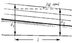
Рис. 126. Течение в русле с уклоном
