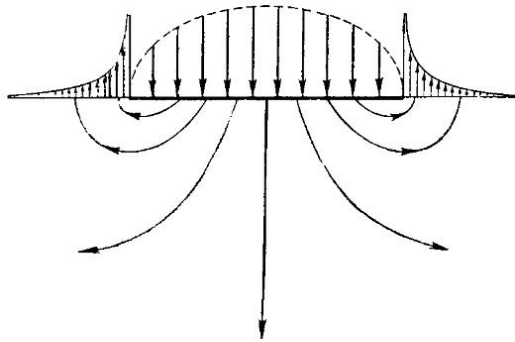
Рис. 269. Распределение давления вдоль ширины плоского дна при погружении в воду
