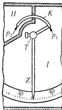
Рис. 16. Прецизионный манометр Рейхардта
